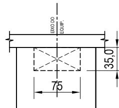
PLANTA P/ EQUIP. DA COBERTURA
