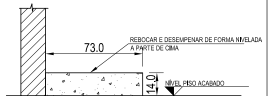
CORTE TRANSVERSAL
