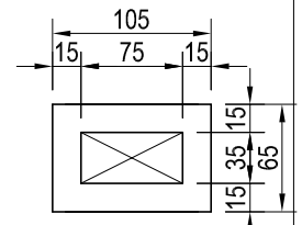
MURETA P/ RUFO DE EQUIP. DA COBERTURA
