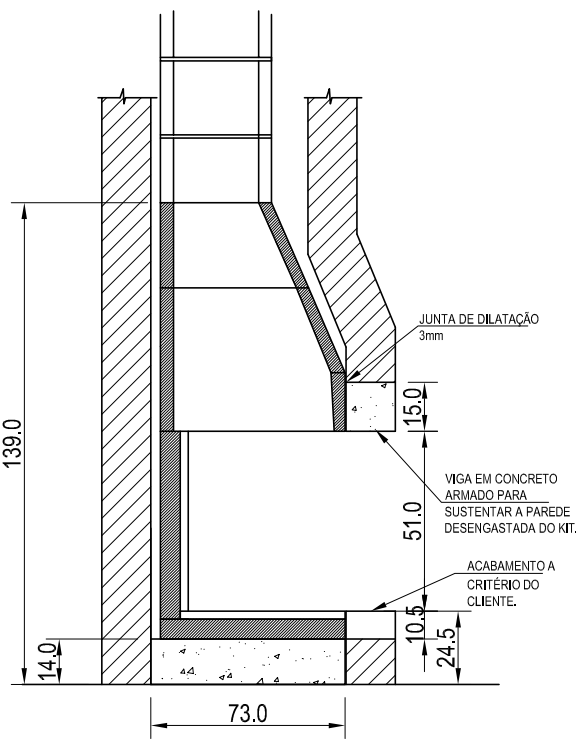
CORTE ACABADO
