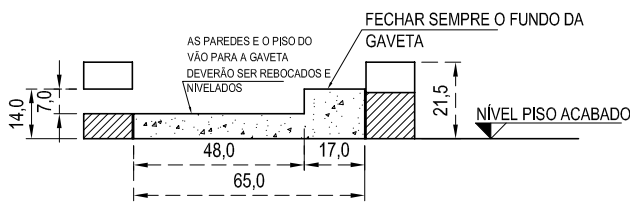
CORTE TRANSVERSAL OBS: EXECUTAR A BASE NIVELADA E ESQUADREJADA, POIS SERÁ A REFERÊNCIA PARA A MONTAGEM DO KIT.
