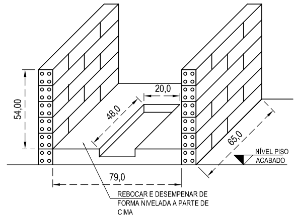
PERPECTIVA DA BASE PARA KIT
